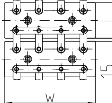
VGM 1000
